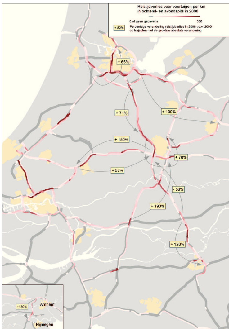
Figuur 4.1 Reistijdverlies op het hoofdwegennet in en rond de Randstad in 2008 en trajecten met de grootste verandering tussen 2000 en 2008 Bron: DVS
