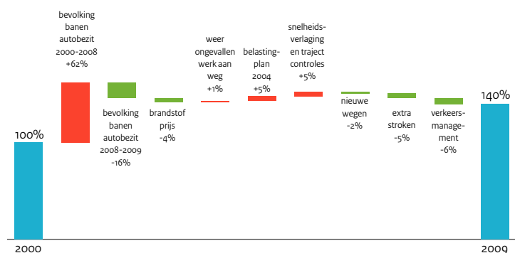
Figuur 4.3 Verklaring toename reistijdverlies door files en vertraagde afwikkeling (ten opzichte van referentiesnelheid 100 km/uur) op het hoofdwegennet 2000-2009.
