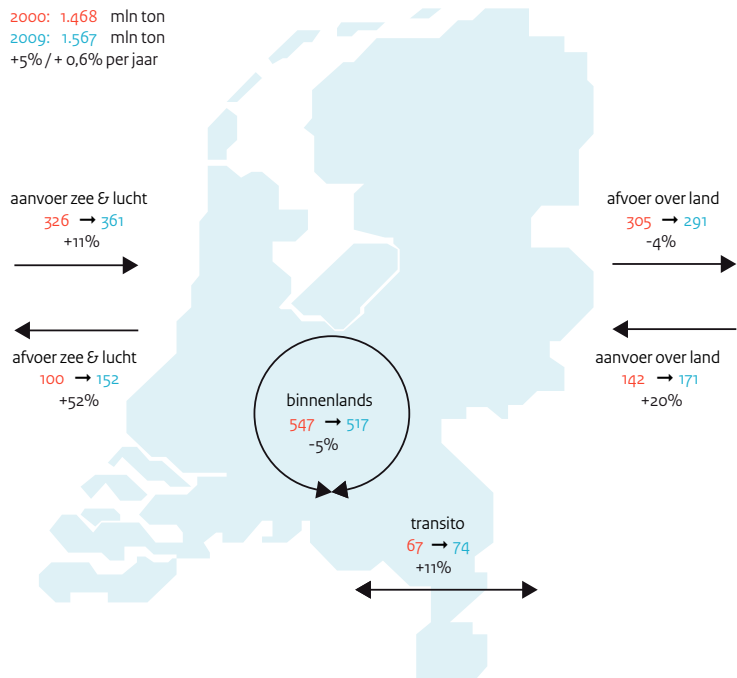
Figuur 3.1 Goederenvervoerstromen in Nederland in 2000 en 2009 (in miljoen ton) Bron: CBS/NEA, bewerking KIM
