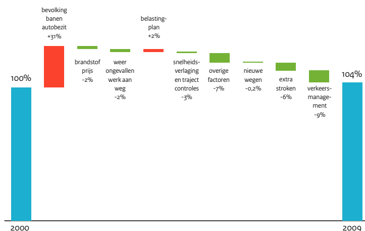
Figuur 4.8 Verklaring ontwikkeling onbetrouwbaarheid op het hoofdwegenet 2000-2009 (Randstad en aansluitende wegen) Bron: Berekening KiM
