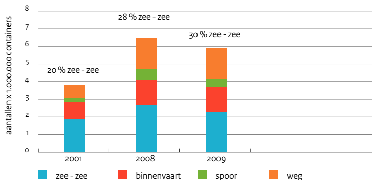
Figuur 3.3 Ontwikkeling modal split in het achterlandvervoer van containers in de Rotterdamse haven (in miljoen containers) Bron: HbR, 2010
